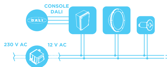
Schema Convertitore DALI - OC
